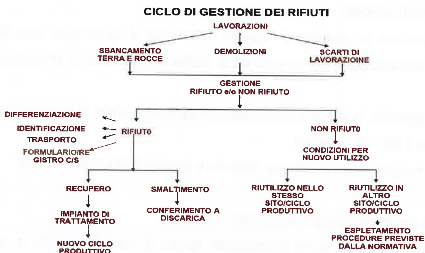
Schema 4 – Il ciclo di gestione dei rifiuti
